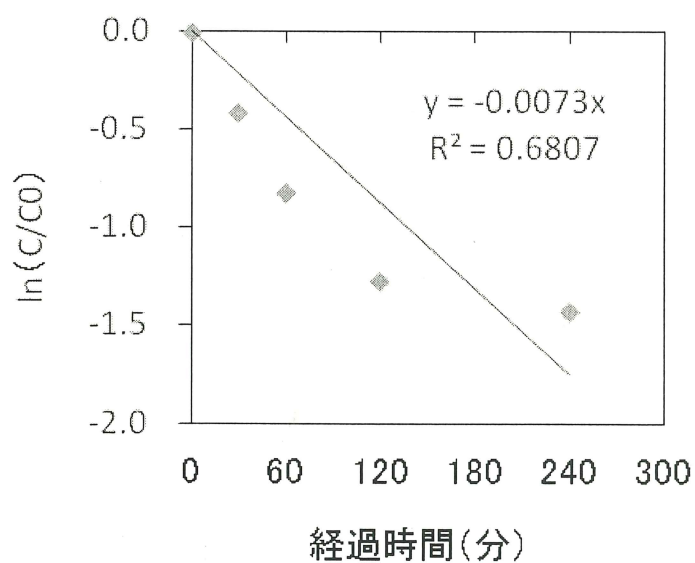
図 1 経過時間と \ln(C/C_0) との関係
