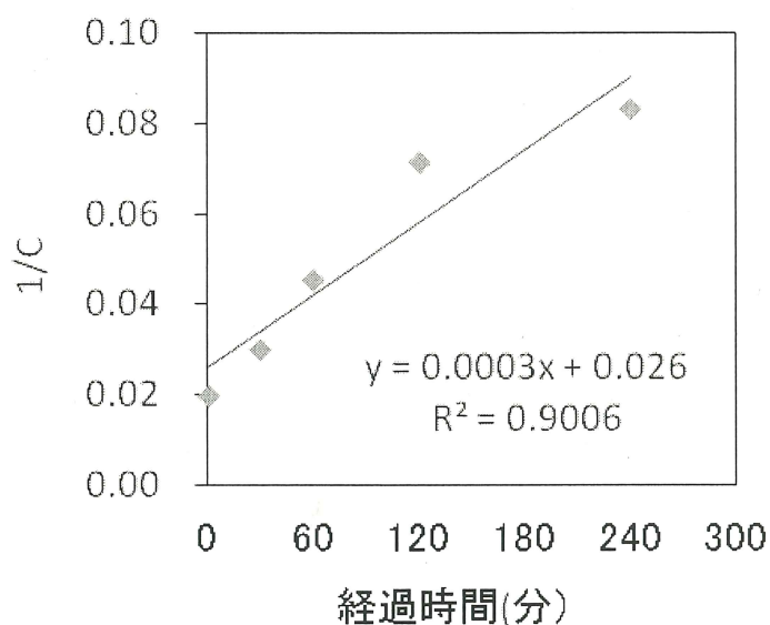
図 2 経過時間と 1/C との関係
